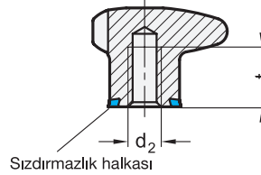
Sızdırmazlık halkası
